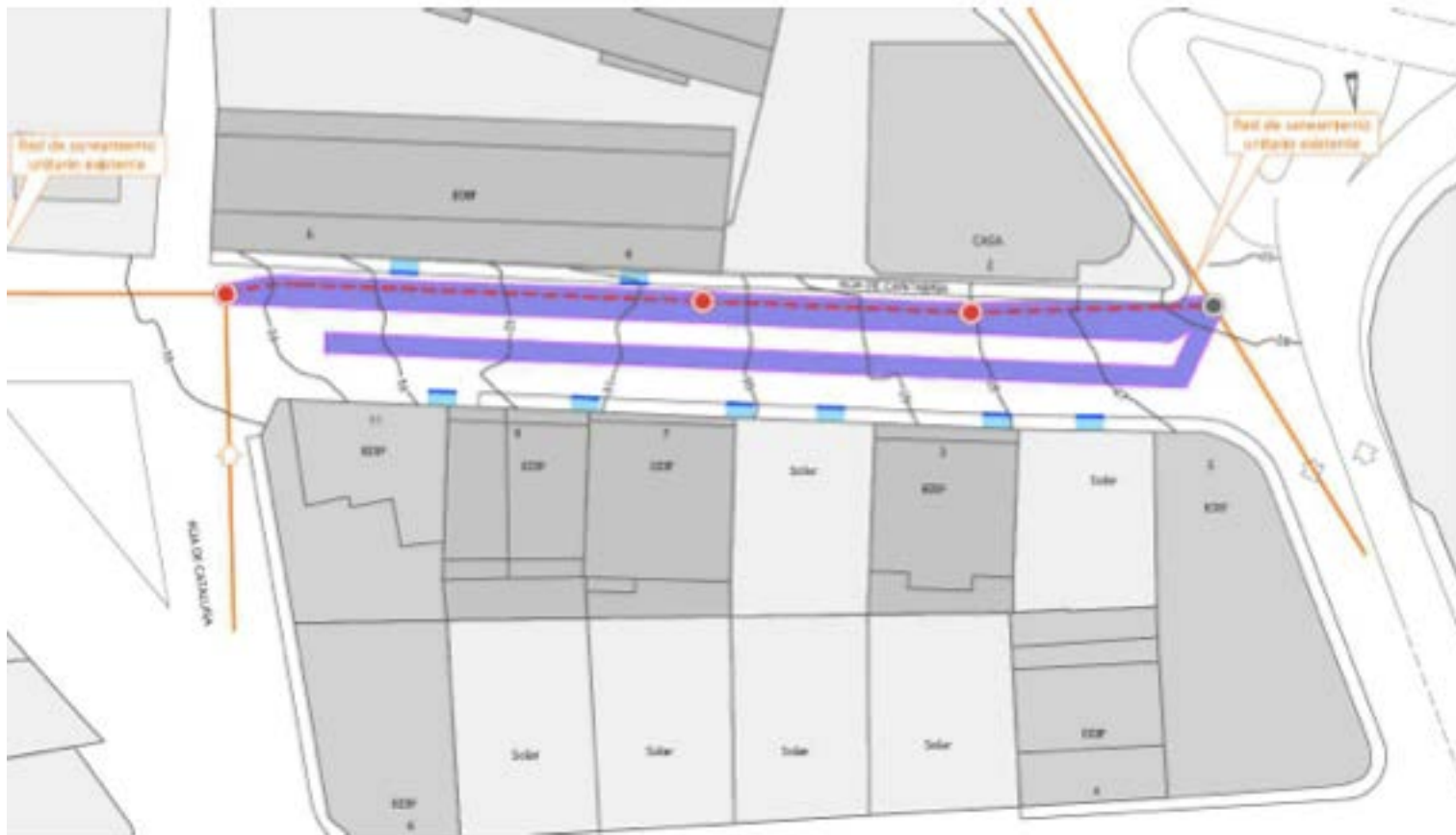
Planta de actuaciones previas (retirada de colector y pozos y demolición de pavimentos)
