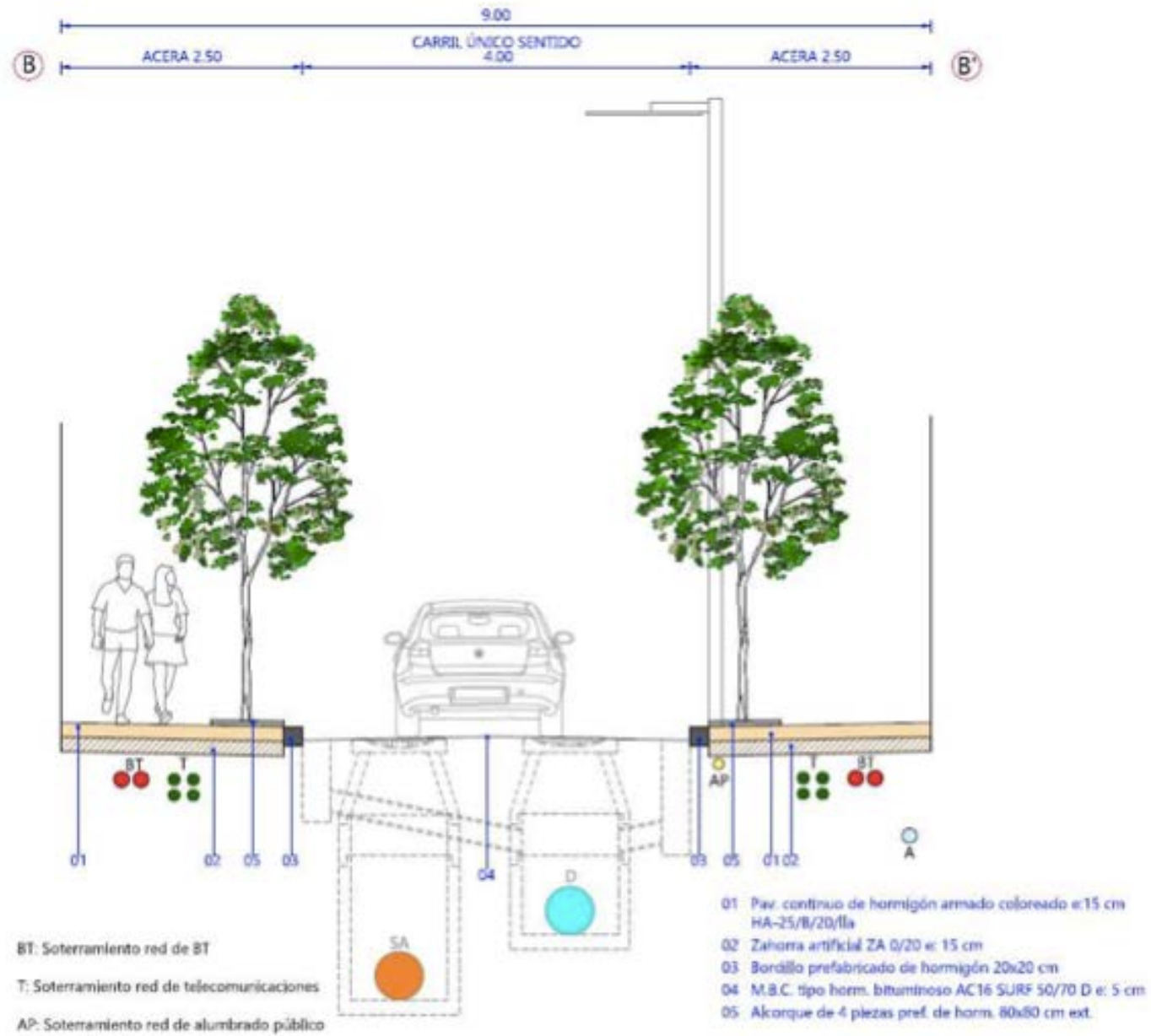
Modelo de actuación en rúas con único sentido de circulación
