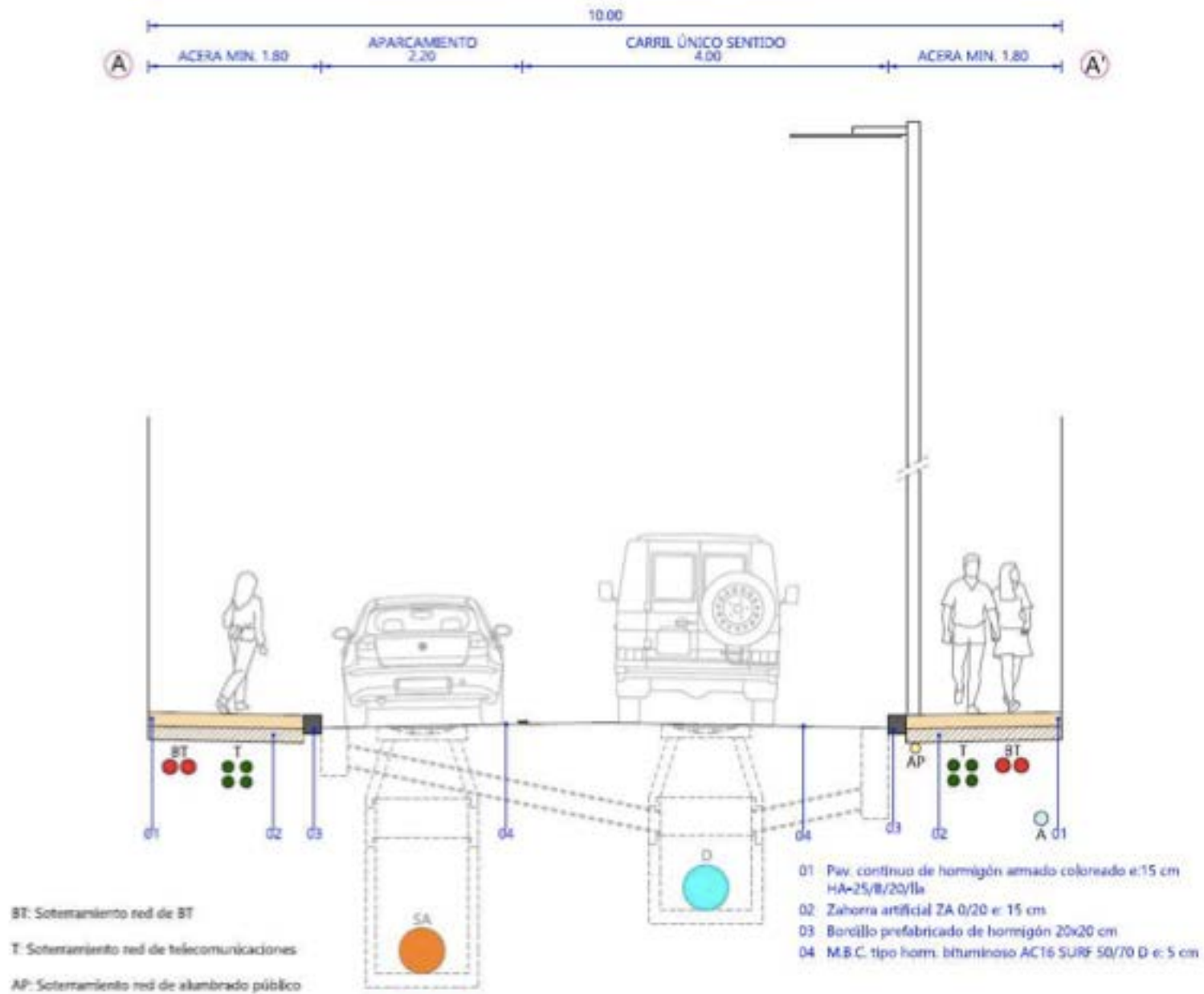
Modelo de actuación en rúas con dobre sentido de circulación
